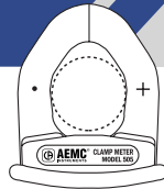
MODELO 505 Abertura de la pinza: 30 mm (1,18 pulg.) Tamaño del conductor: un cable de 500 kcmil
