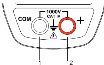
Figura 4 : los bornes
