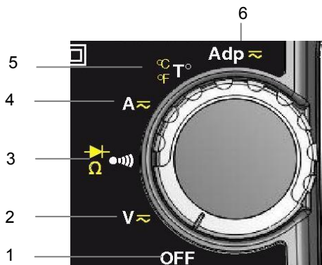
Figura 2 : el conmutador
