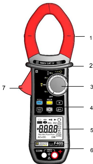
Figura 1 : la pinza multimétrica F405
