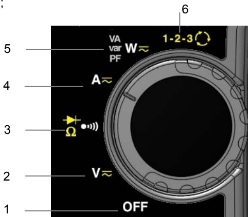
Figura 2 : el conmutador
